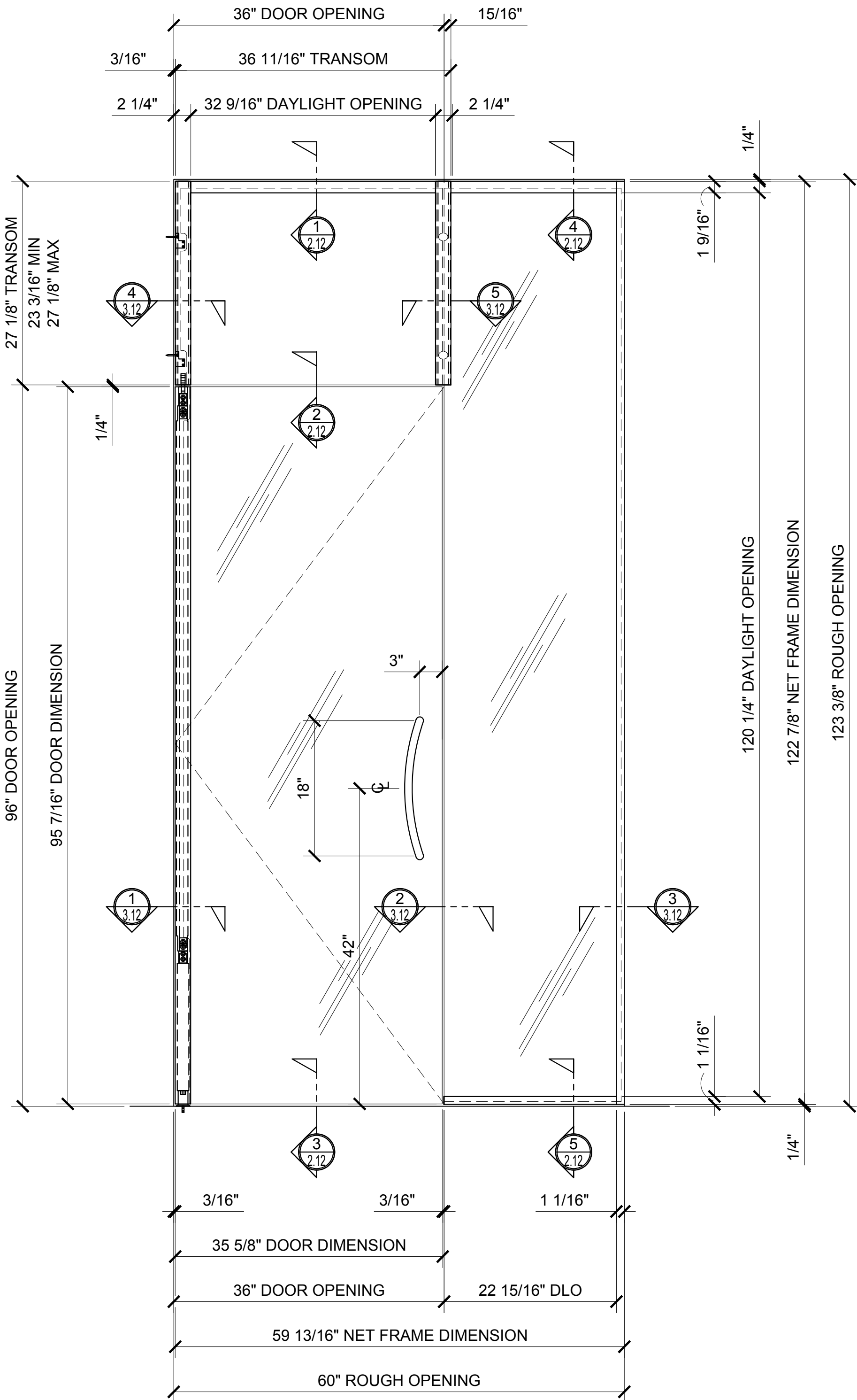
2 ELEVATION
