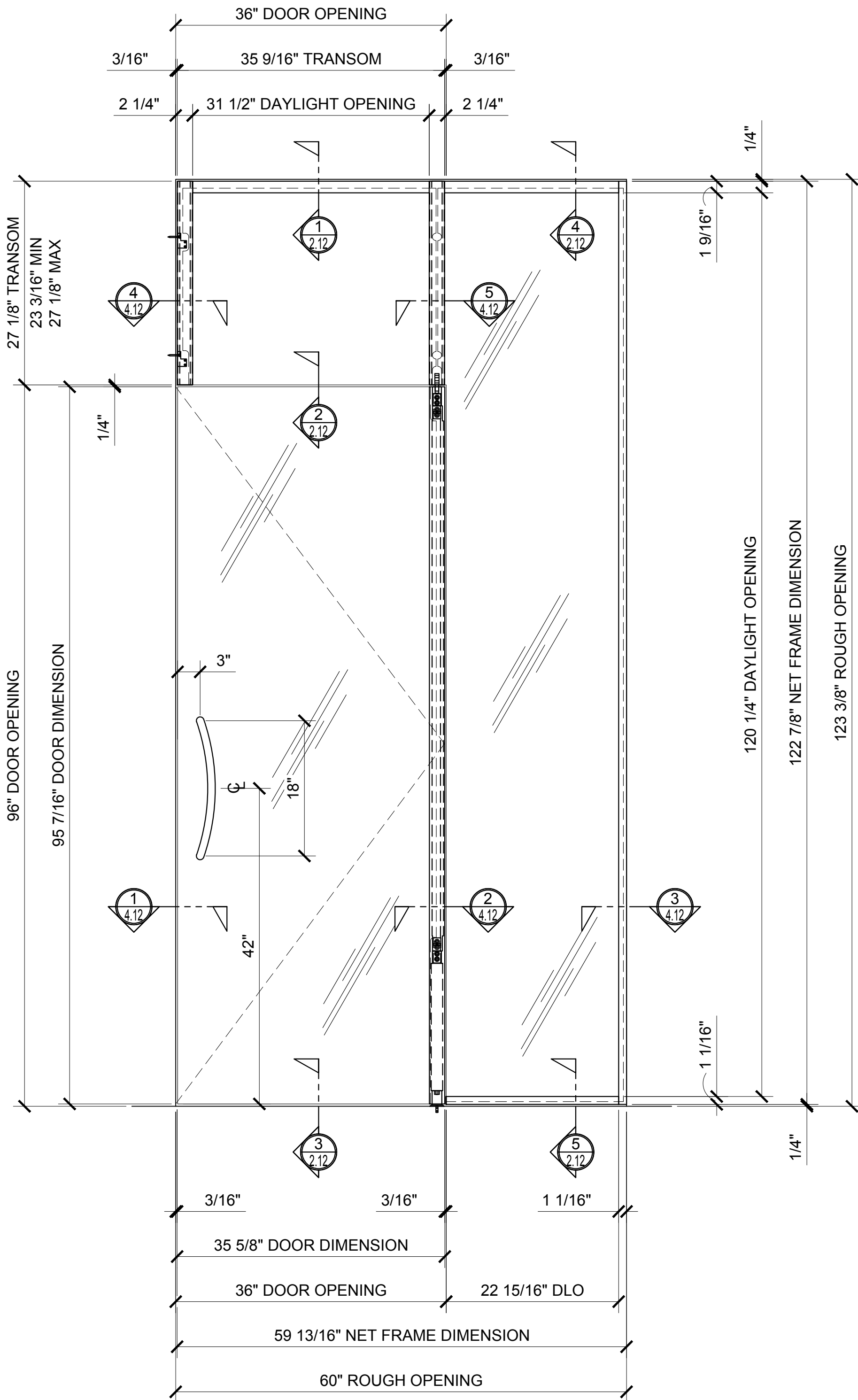
4 ELEVATION
