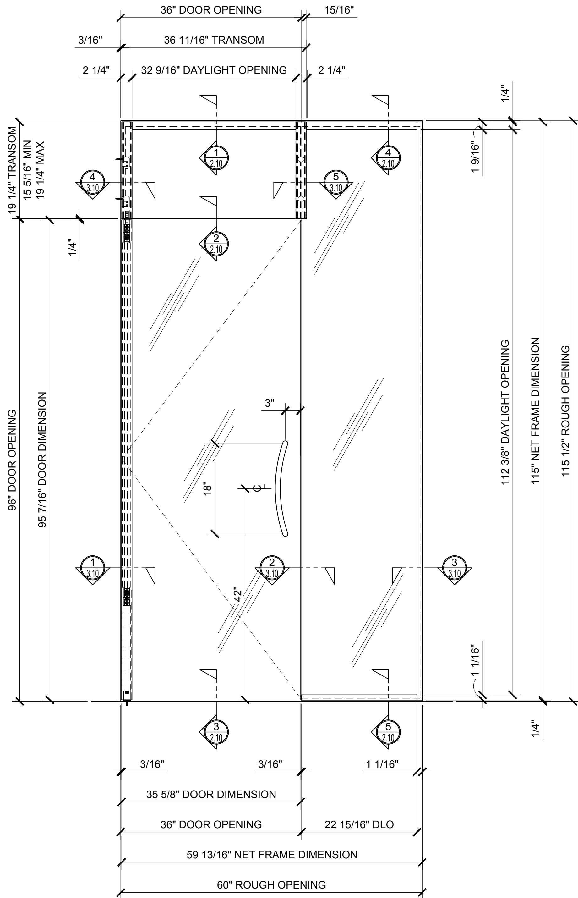
2 ELEVATION
