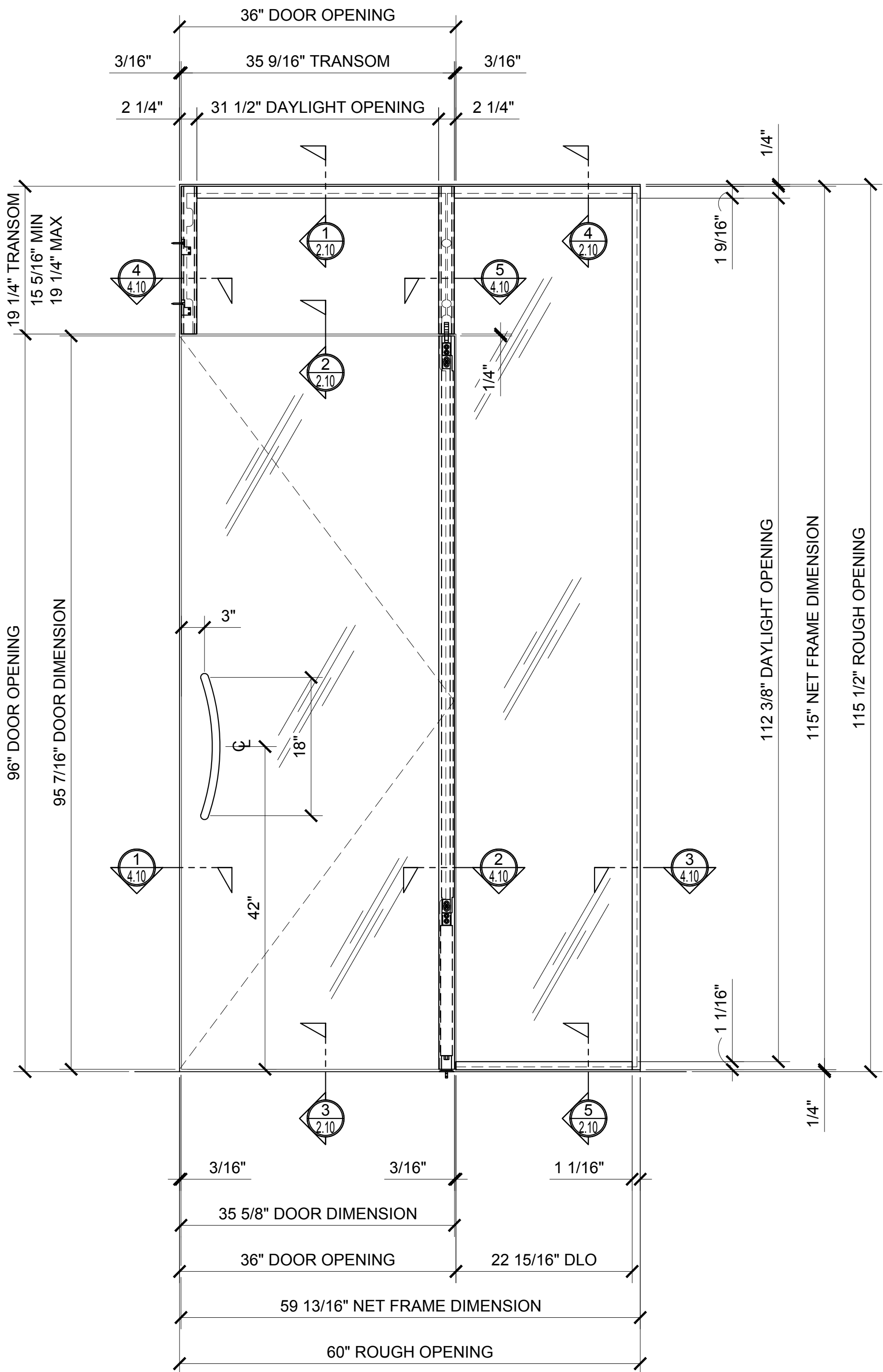
4 ELEVATION
