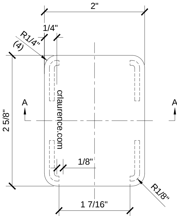
CAP PLAN
