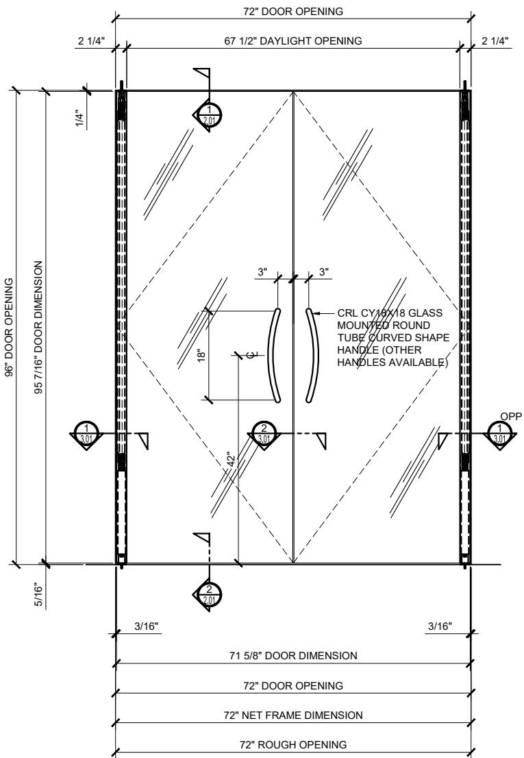
② ELEVATION
