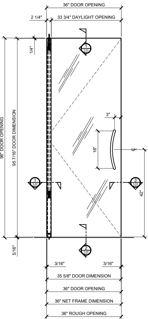
④ ELEVATION
